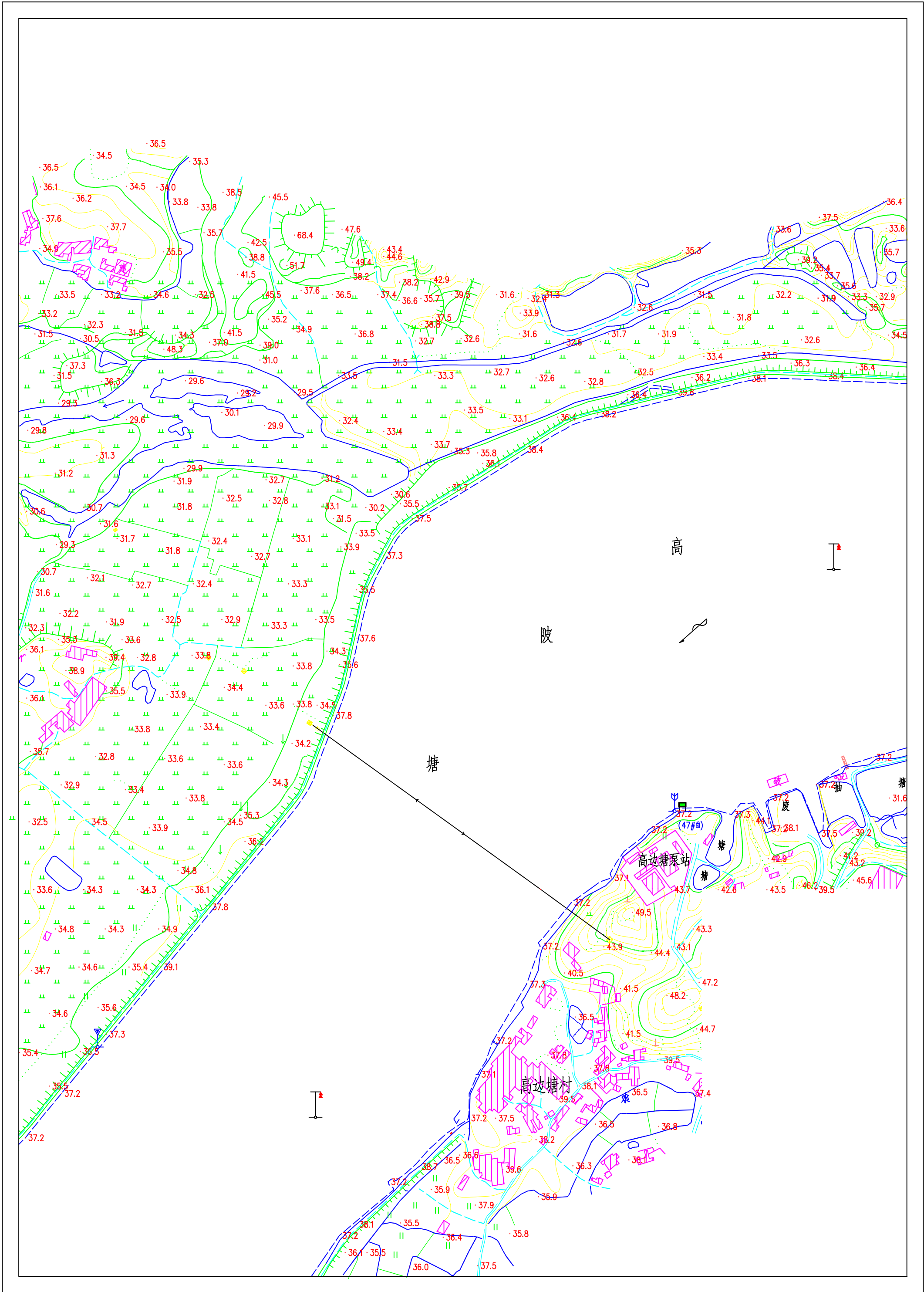
北江110kV石龙线维修施工期航标配布示意图
