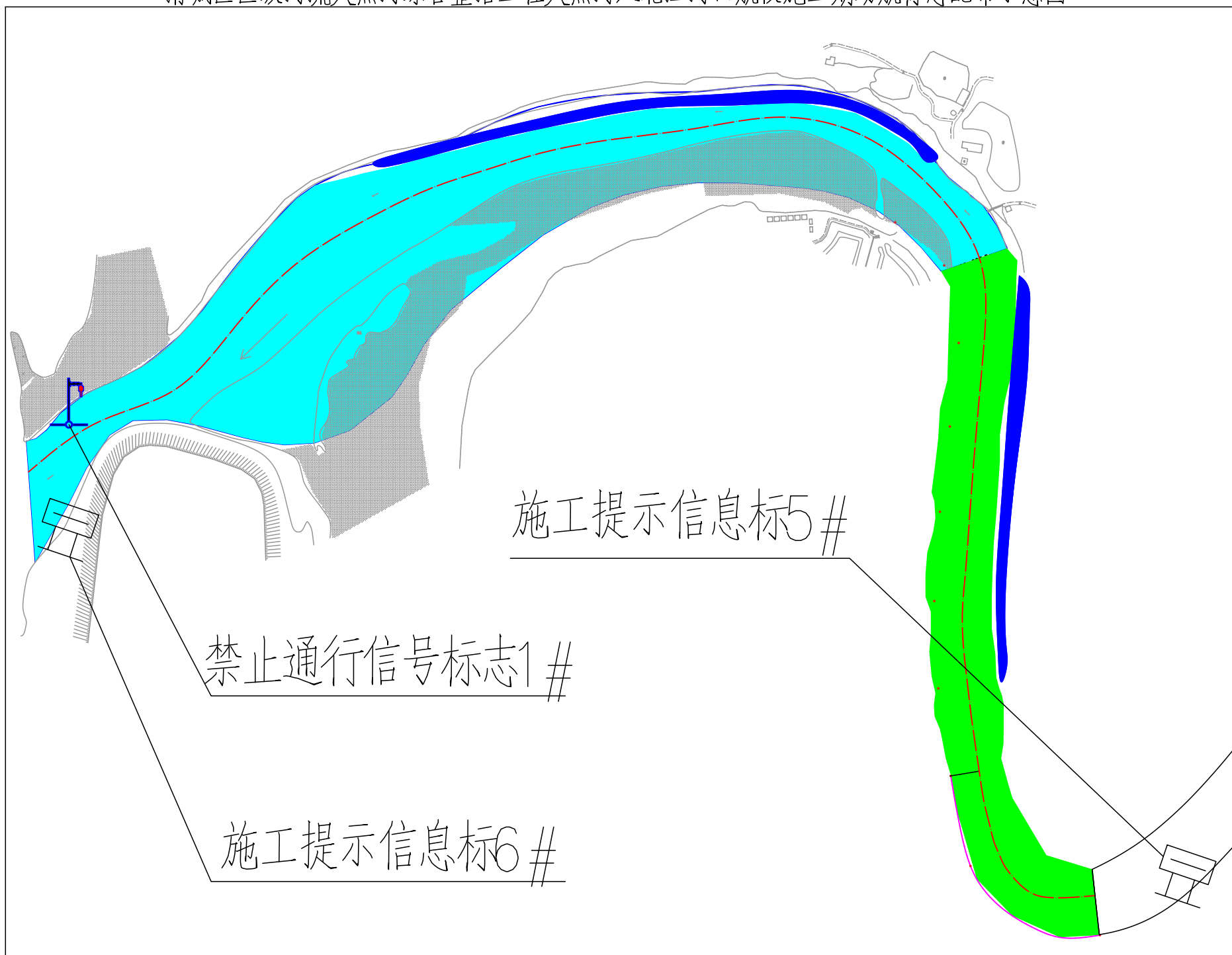
清城区区级河流大燕河综合整治工程大燕河入北江河口航段施工期助航标志配布示意图
