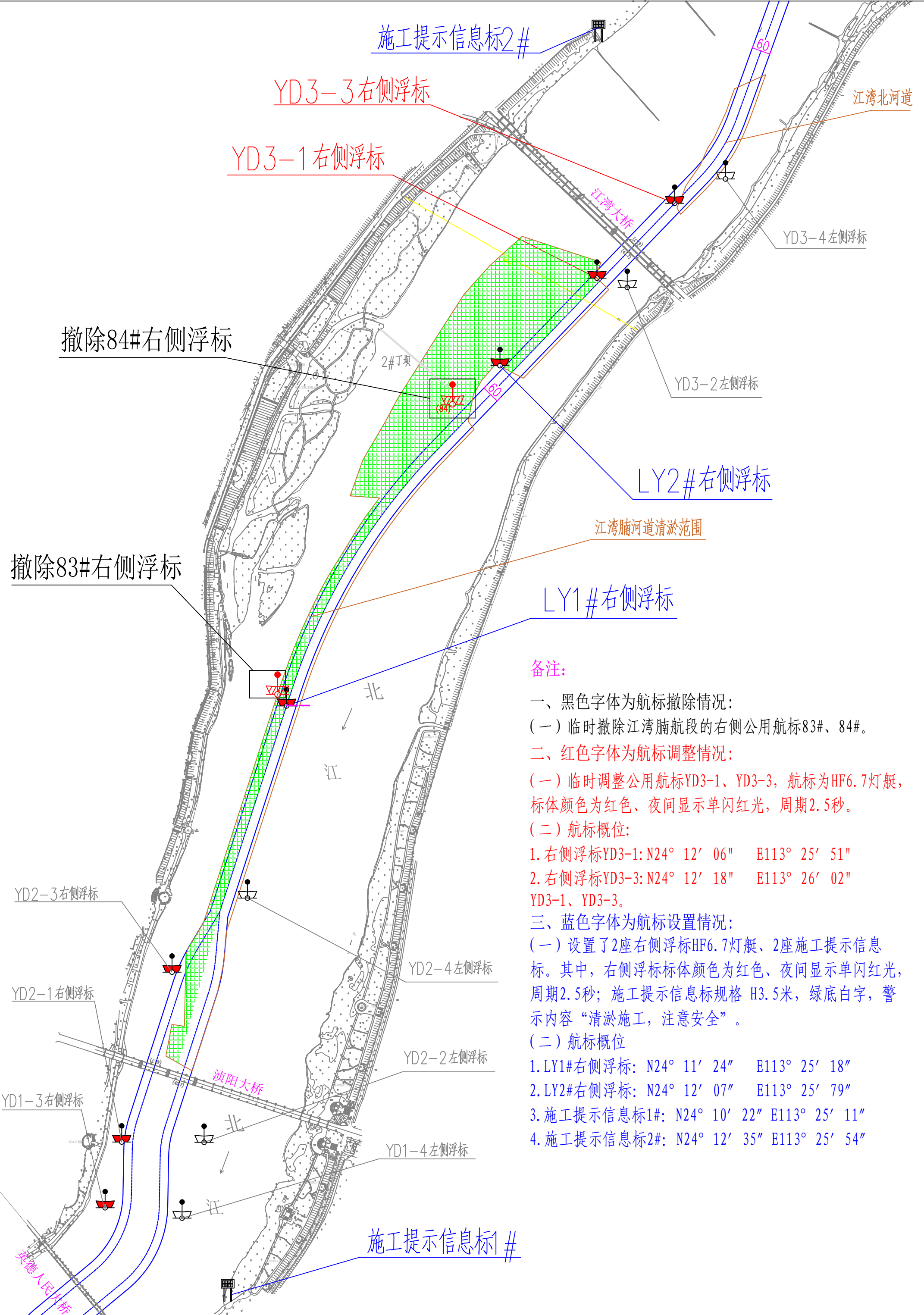
北江干流英德龙尾山至浚阳大桥段河道清淤工程江湾肱航段右侧施工期助航标志配布示意图
