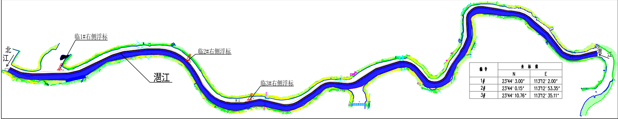
清远市清城区区级河流高田河、滘江河综合整治工程施工期助航标志配布示意图
