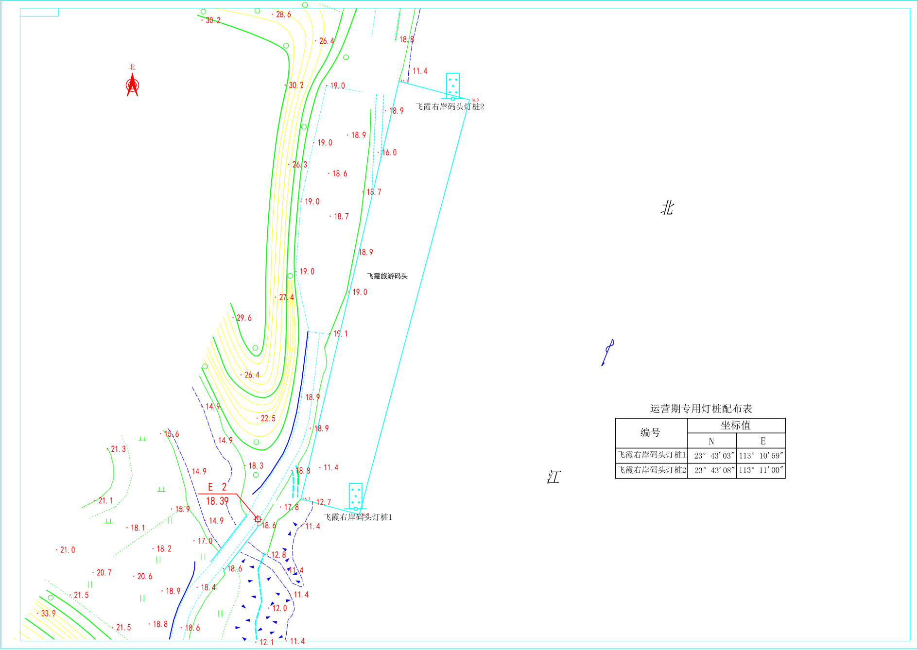
飞霞旅游码头营运期航标配布示意图
