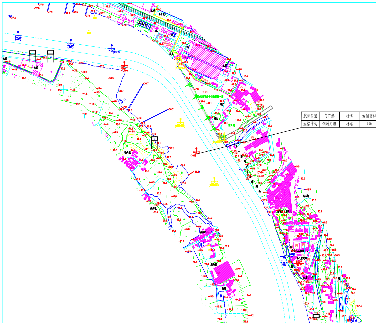
北江乌石港河段航道航标配布示意图
